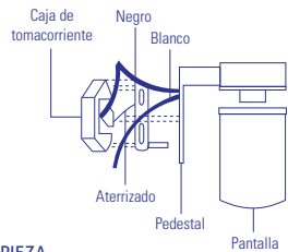
DIAGRAMA ELÉCTRICO (B) Cable blanco: Neutro (N) Cable negro: Línea (⊕) Cable de cobre: Tierra
